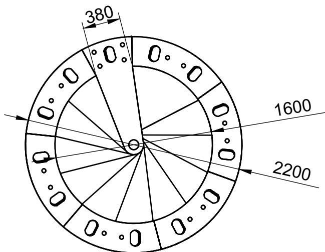
Вид сверху
